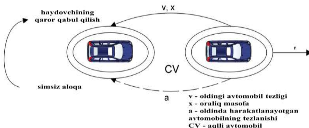
1-rasm. Ulangan transport vositasi uchun ergashib harakatlanish modelining konfiguratsiyasi.
